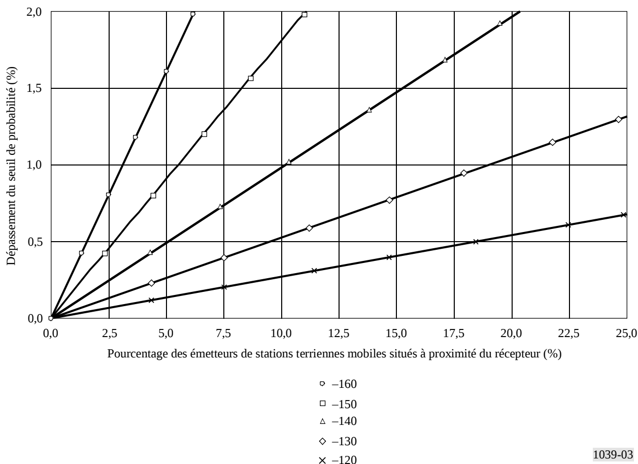
FIGURE 3 Probabilité de brouillage
